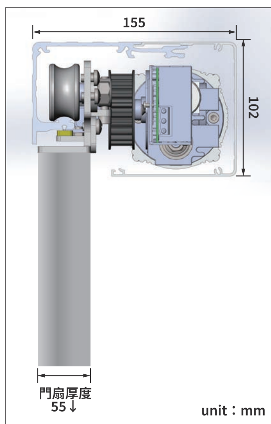
斷面尺寸圖
